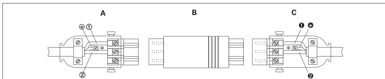
Abb. 4 Anschluss des Steckverbinders
