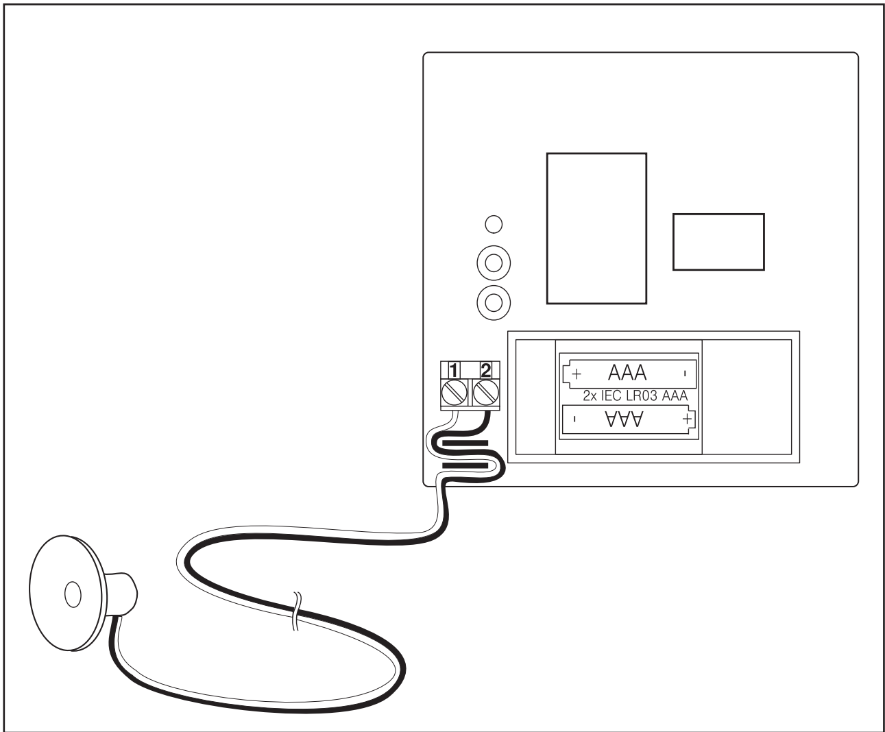
Abb. 2 Anschluss des Dämmerungssensors, Einsetzen der Batterien
