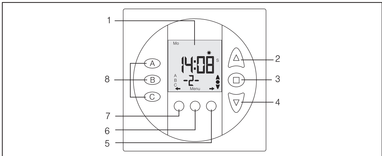
Abb. 4 Bedien- und Anzeigeelemente
