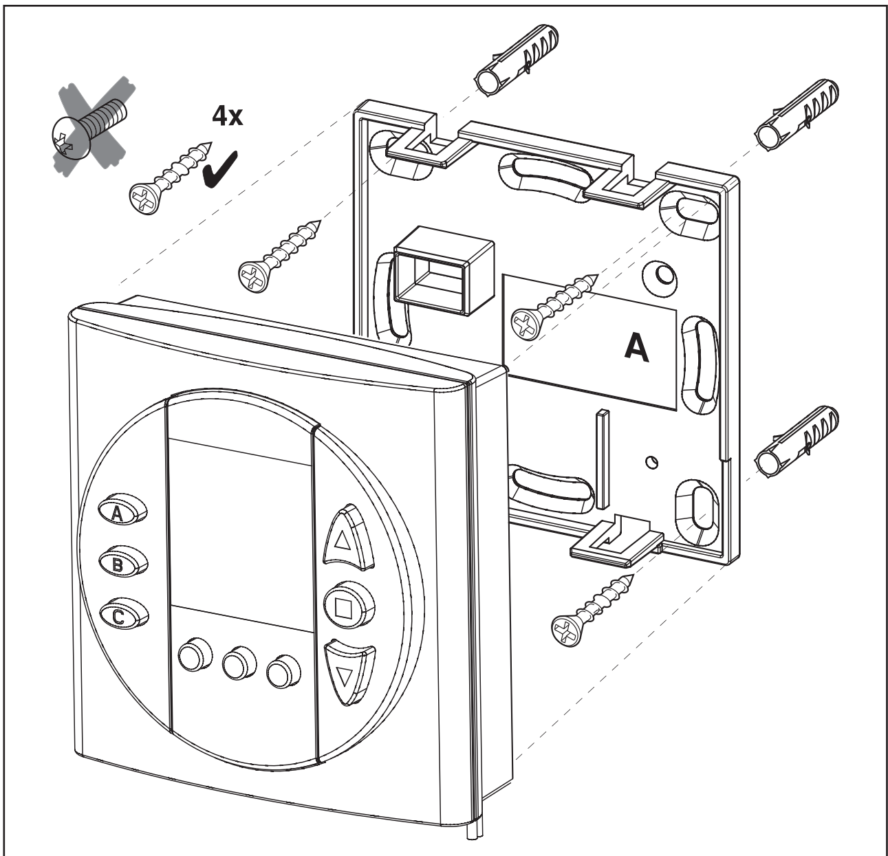
Abb. 1 Wandmontage
