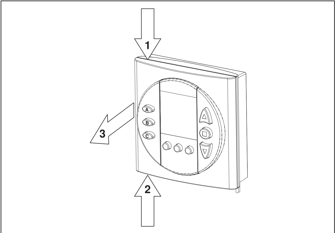
Abb. 3 Demontage
