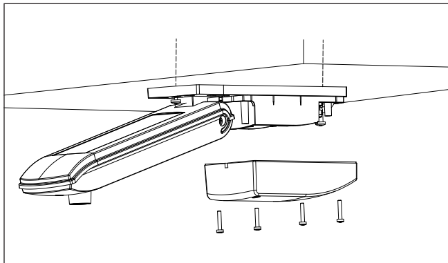
Abb. 5 Deckenmontage
