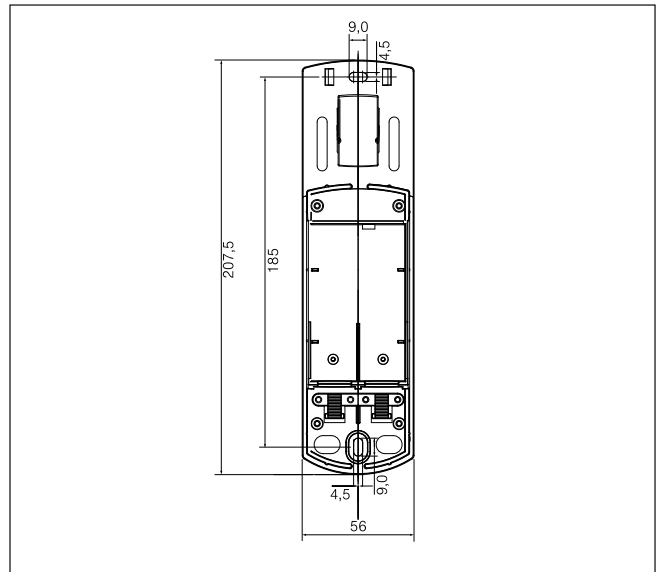
Abb. 3 Abmessungen
