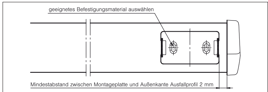
Abb. 4 Montage des WMS Windsensors bei anderen Markisentypen
