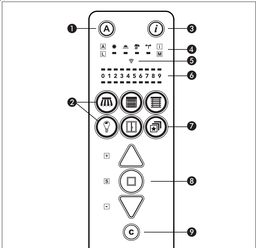
Abb. 7 Bedienfeld des WMS Handsender comfort
