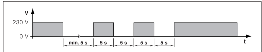
Abb. 9 PowerUp am WMS Zwischenstecker
