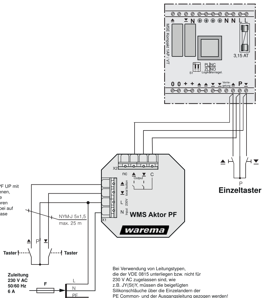
Abb. 2 Anschlussbeispiel WMS Aktor PF UP
