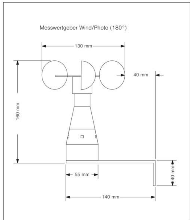
Abb. 3 Abmessungen
