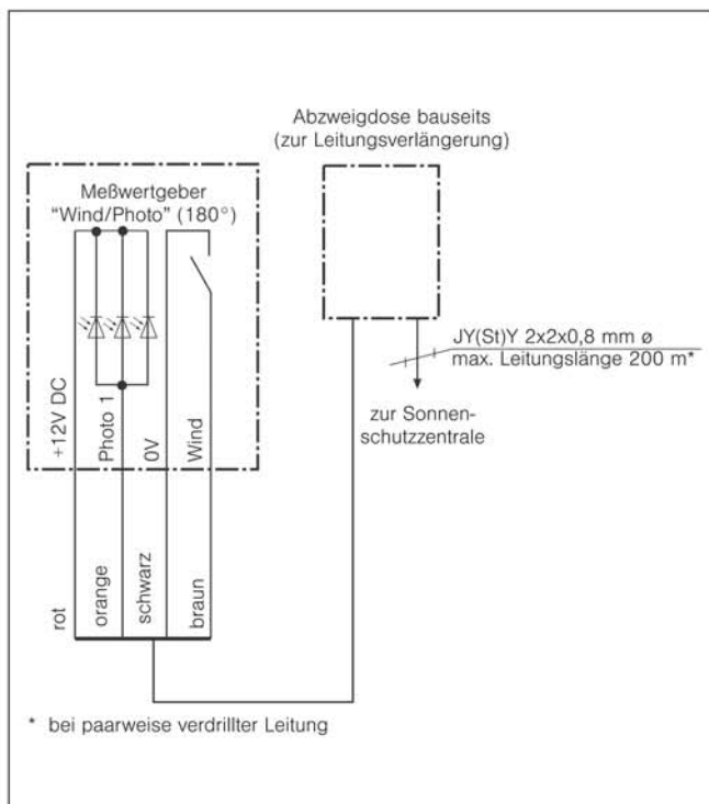
Abb. 2 Anschlussplan
