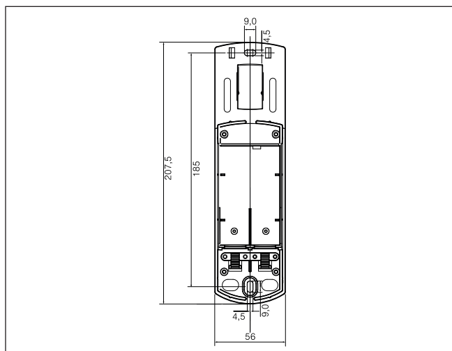
Abb. 3 Abmessungen
