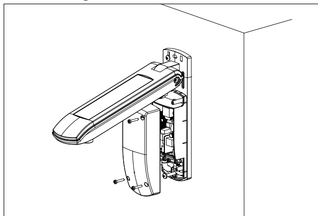
Abb. 4 Wandmontage
