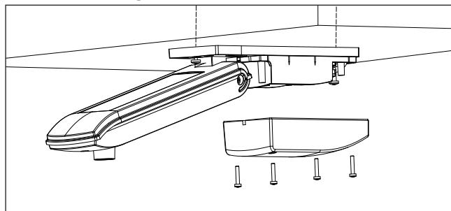
Abb. 5 Deckenmontage
