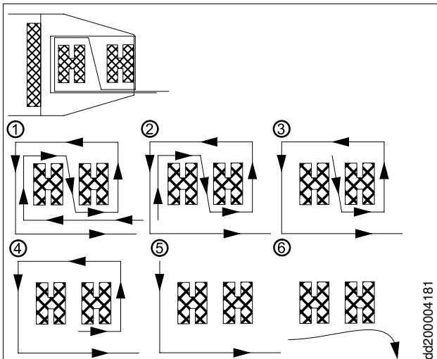
Abb. 2: Zugband entfernen
