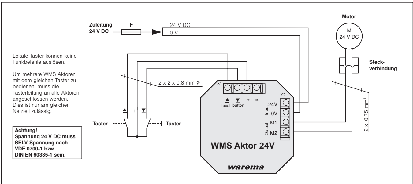
Abb. 2 Anschlussbeispiel Motor
