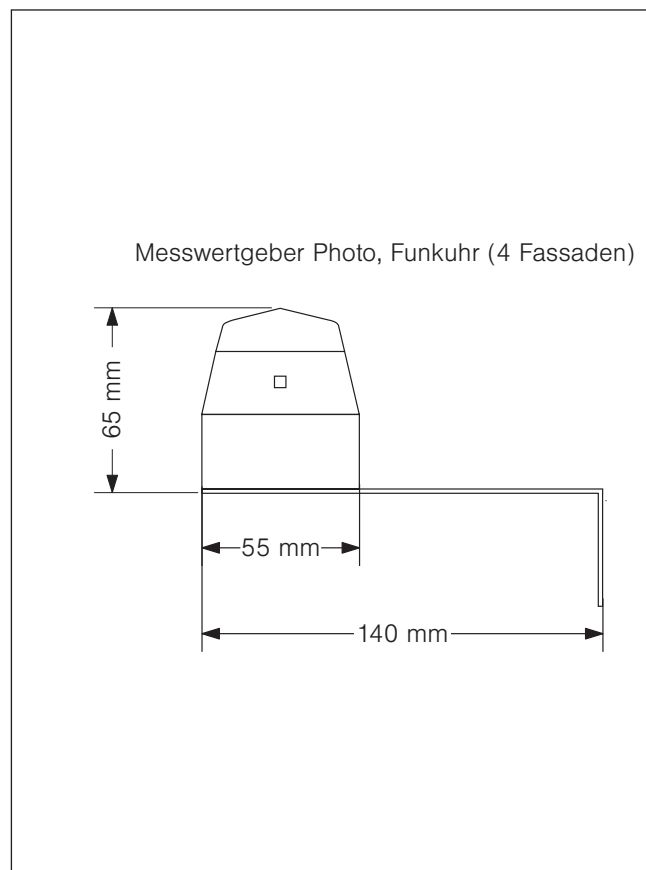
Abb. 4 Abmessungen
