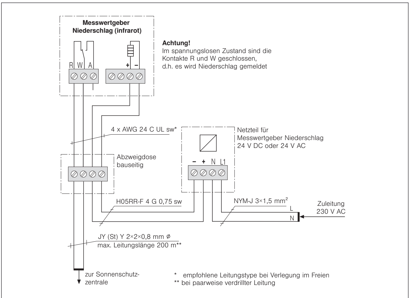
Abb. 6 Anschlussplan
