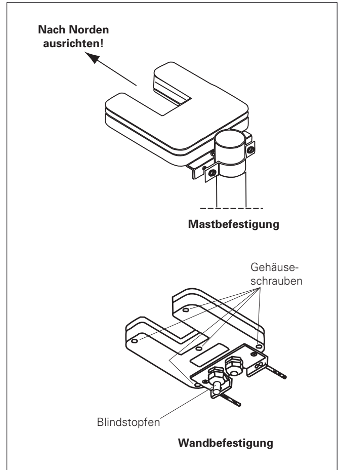
Abb. 7 Montagehinweise
