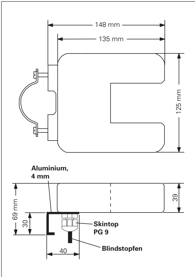
Abb. 5 Abmessungen
