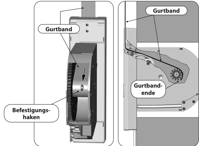
Gurtbandverlauf im RolloTron Comfort DuoFern
