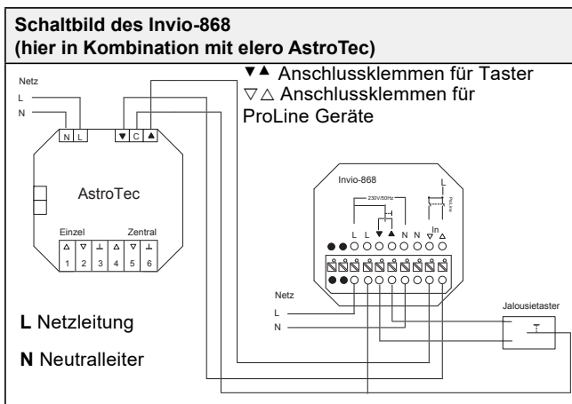
Fig. 3 Schaltbild zum Anschluss des Invio-868 an vorhandene elero Steuerungskomponenten (hier am Beispiel AstroTec)
