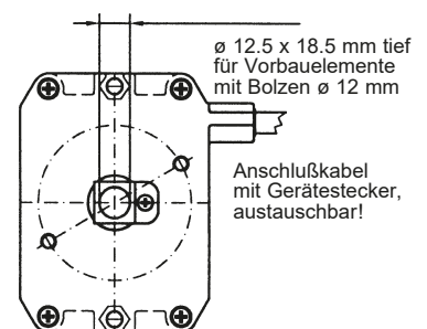
Kabelaustritt hinten
