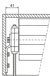
Wandanker 13 301.0801
