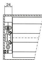
Vorbau- Element
