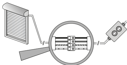
Fig. 5 Anschluss für Montagekabel
