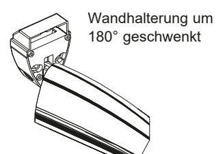
Wandhalterung um 180^\circ geschwenkt Mast- und Eckbefestigung Sonderzubehör (Artikel-Nr. 24 269.0201)
